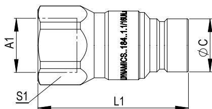
Male Quick Coupler size 12,7 (1/2") or 19,1 (3/4") Schnellverschluss-Männchen Größe 12,7 (1/2") oder 19,1 (3/4") Raccord rapide mâle taille 12,7 (1/2") ou 19,1 (3/4")
