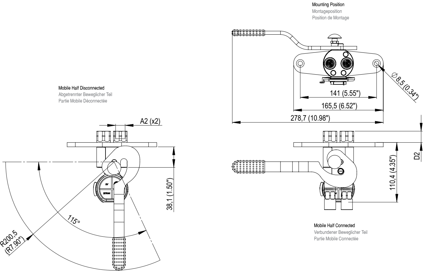
Fixed Half / Fester Teil / Partie Fixe
