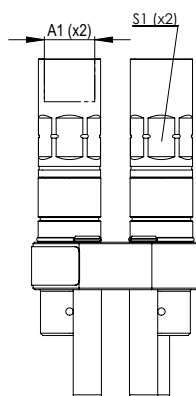
Mobile Half / Bewegliches Teil / Partie Mobile
