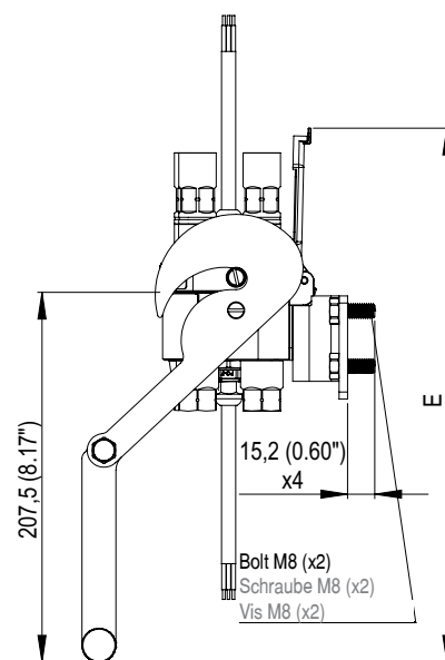
Mobile Half Connected Verbundener Beweglicher Teil Partie Mobile Connectée
