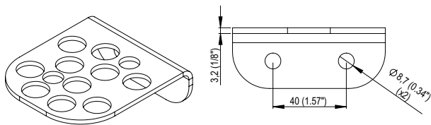
Docking for Mobile Half Unterstützung für Bewegliche Teile Support pour Partie Mobile
