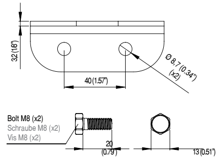
Docking for Mobile Half Stütze für den Beweglichen Teil Support pour la Partie Mobile
