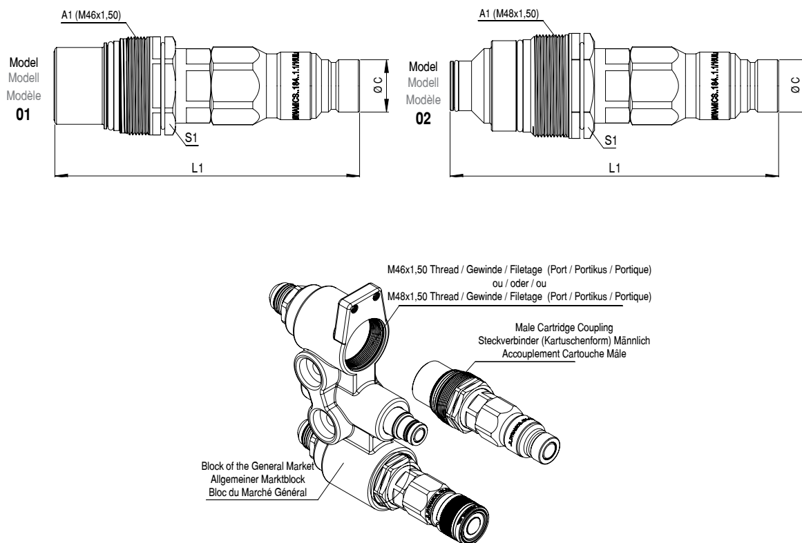
Male Cartridge Coupler / Steckverbinder (Kartuschenform) Männlich / Accouplement Cartouche Mâle
