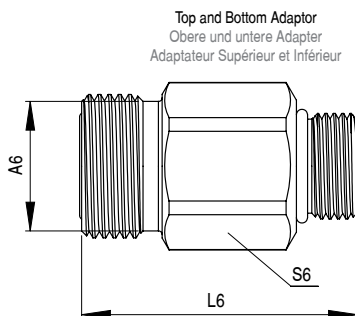
Top and Bottom Adaptor / Obere und untere Adapter / Adaptateur Supérieur et Inférieur
