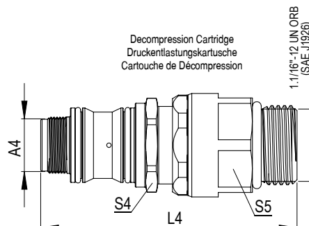
Male Quick Coupler Top Line / Schnellverschluss-Männchen der Leitung / Raccord Rapide Mâle de La Ligne
