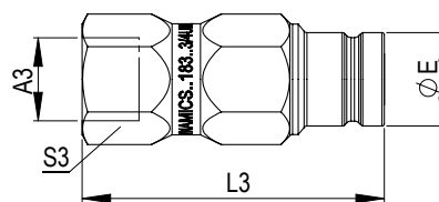
Male Quick Coupler size 9,5 (3/8") - DRAIN LINE Schnellverschluss-Männchen Größe 9,5 (3/8") - DRAIN LINE Raccord rapide mâle taille 9,5 (3/8") - DRAIN LINE
