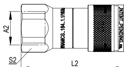
Female Quick Coupler size 12,7 (1/2") or 19,1 (3/4") Schnellverschluss-Weibchen Größe 12,7 (1/2") oder 19,1 (3/4") Raccord rapide femelle taille 12,7 (1/2") ou 19,1 (3/4")
