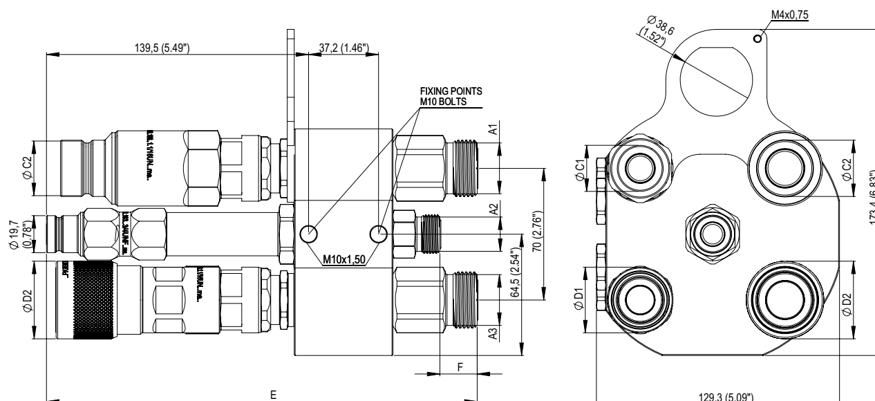
Decompression Block Coupler / Block Mit Entlüftungsventilen / Bloc Avec Raccords à Soupape de Décompression
