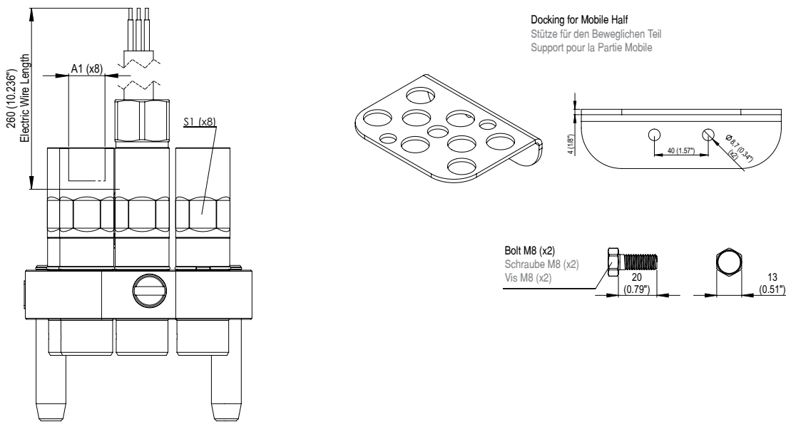
Mobile Half / Bewegliches Teil / Partie Mobile
