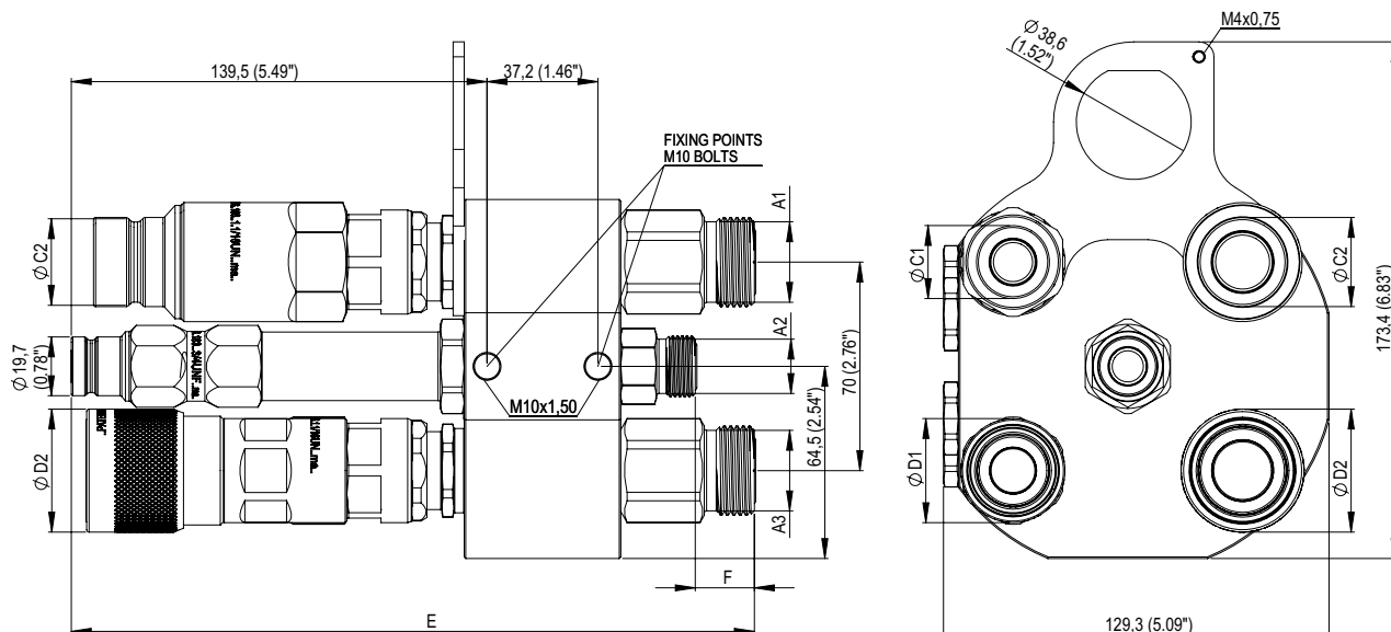
Bloco com Engates com Válvula de Despressurização / Bloque de Acoplamiento con Válvula de Despresurización / Decompression Block Coupler
