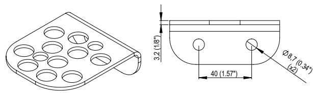
Apoio para Parte Móvel Soporte para Piezas Móviles Docking for Mobile Half
